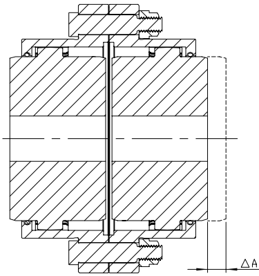
Desalineamiento de los Ejes
