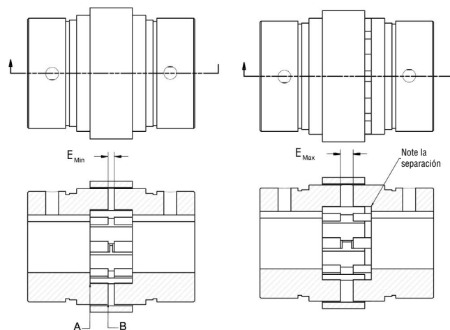
Figura 2. Go-Flex® de Martin - Alineamiento de la Maza al Eje Ve la página C-77 para las Tolerancias de Desalineamiento.
