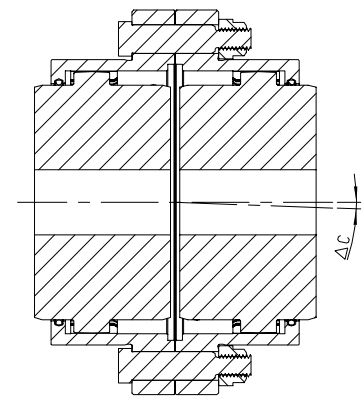
Desalineamiento Angular
